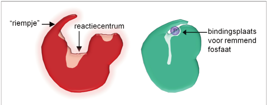
Figuur 33: Links: De actieve vorm van het SRC-eiwit. Het reactiecentrum is open. Rechts: De inactieve vorm, met een fosfaat (P) dat het riempje vastzet waarmee SRC wordt dichtgebonden. Die P wordt afgeknipt om SRC te activeren. In het kankerwekkende SRC kan deze P er door mutatie niet aangezet worden, wordt SRC niet dichtgebonden en daardoor te gemakkelijk geactiveerd.
